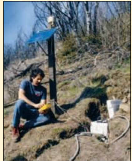
▲ Figura 15.C Prueba de un sistema de radioteleetría alimentado con energía solar para la transmisión a distancia de datos de un deslizamiento en tiempo real. En las zonas de deslizamiento controladas a distancia, el movimiento del suelo y las presiones de las aguas subterráneas se miden cada segundo. La cantidad del movimiento descendente es registrada por extensómetros que pueden detectar la tensión o el acortamiento del suelo. Las vibraciones del suelo se controlan mediante geófonos enterrados en el interior de los deslizamientos. Las condiciones de las aguas subterráneas en el interior de los deslizamientos se controlan a través de sensores de la presión del agua de los poros y los pluviómetros in situ registran las precipitaciones. (Foto de Mark Reid/U. S. Geological Survey.)
