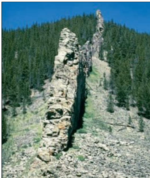
▲ Figura 5.17 La estructura vertical del fondo es un dique, que es más resistente a la meteorización que la roca circundante. Este dique se encuentra al oeste de Granby, Colorado, cerca del Arapaho National Forest. (Foto de R. Jay Fleisher.)
