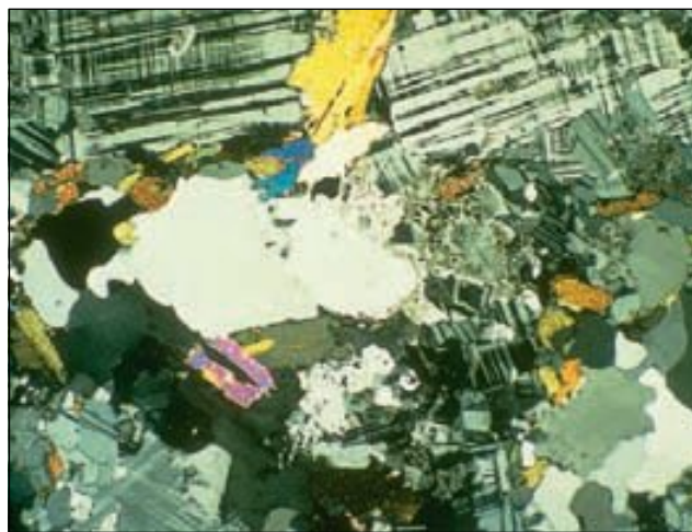
▲ Figura 4.1 A. Vista de cerca de cristales entrecrecidos en una roca ígnea de grano grueso. Los cristales más grandes tienen alrededor de un centímetro de longitud. B. Microfotografía de cristales entrecrecidos en una roca ígnea de grano grueso. (Fotos de E. J. Tarbuck.)
