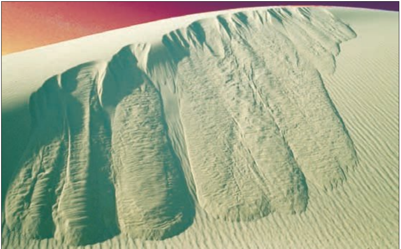
▲ Figura 19.12 Arena descendiendo por la cara de deslizamiento empinada de una duna, en el Monumento Nacional White Sands, Nuevo México. (Foto de Michael Collier.)
