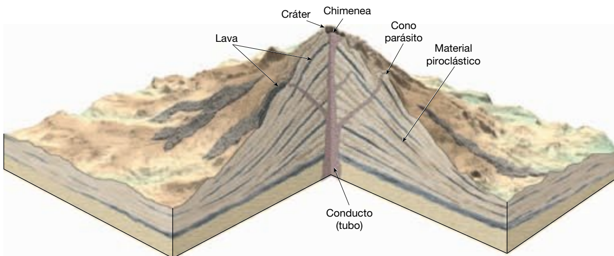
▲ Figura 5.4 Anatomía de un cono compuesto «típico» (en la Figura 5.5 se puede comparar con un volcán en escudo y un cono de ceniza, respectivamente).
