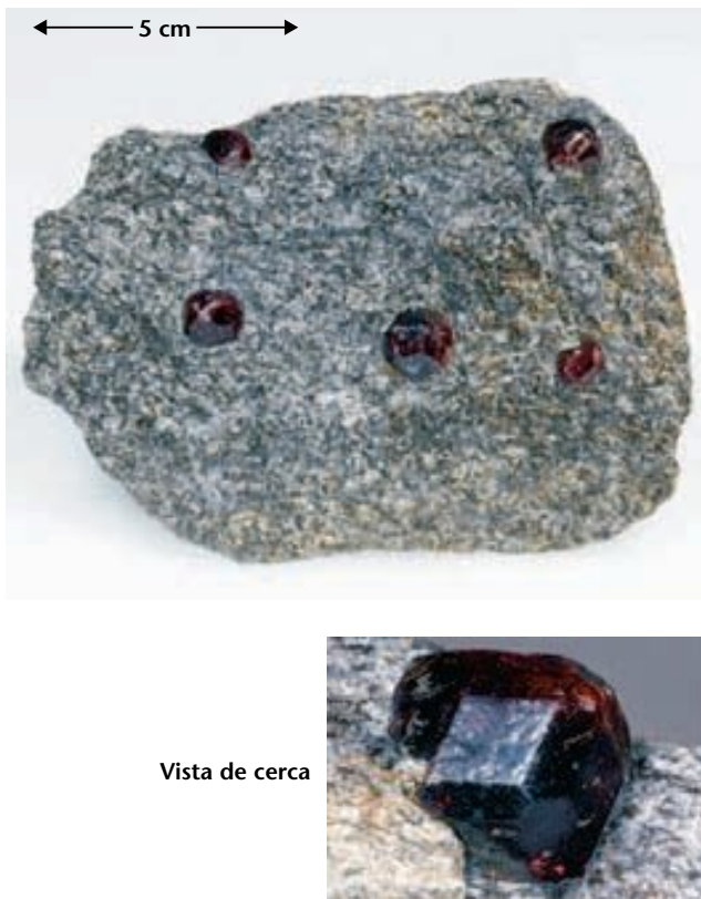
▲ Figura 8.8 Micaesquisto granatífero. Los cristales rojo oscuro del granate (porfidoblastos) están incrustados en una matriz clara de micas de grano fino. (Foto de E. J. Tarbuck.)
