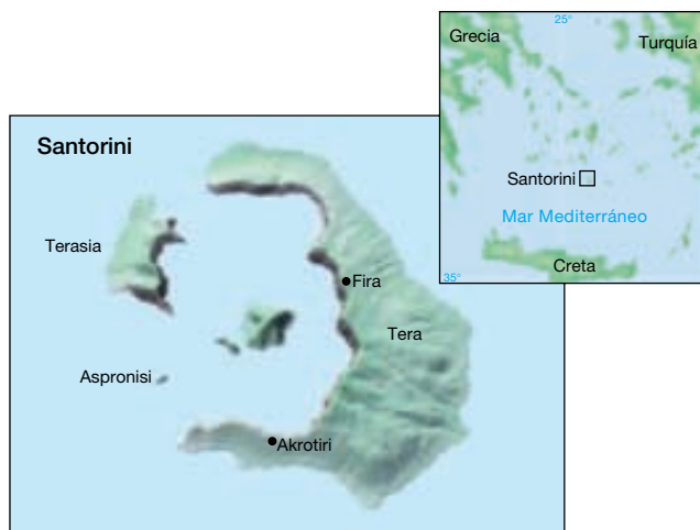
▲ Figura 5.10 Mapa que muestra los restos de la isla volcánica de Santorini después de que la parte superior del cono se hundiera en la cámara magmática vacía tras una erupción explosiva. Se muestra la localización de la población minoica recientemente excavada de Akrotiri. Las erupciones volcánicas durante los últimos 500 años formaron las islas centrales. Pese a la posibilidad de que se produzca otra erupción destructiva, la ciudad de Fira se edificó en los flancos de la caldera.
