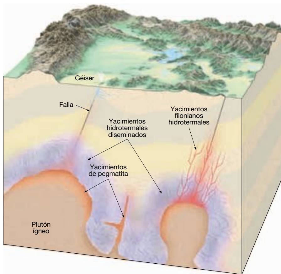
► Figura 21.17 Ilustración que representa la relación entre un cuerpo ígneo y los yacimientos hidrotermales y de pegmatita asociados.
