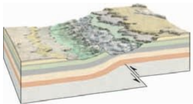
▲ Figura 10.12 Monoclinal. El monoclinal consiste en estratos sedimentarios plegados que fueron deformados por una fractura del basamento. El cabalgamiento de este diagrama se denomina cabalgamiento ciego porque no alcanza la superficie.
