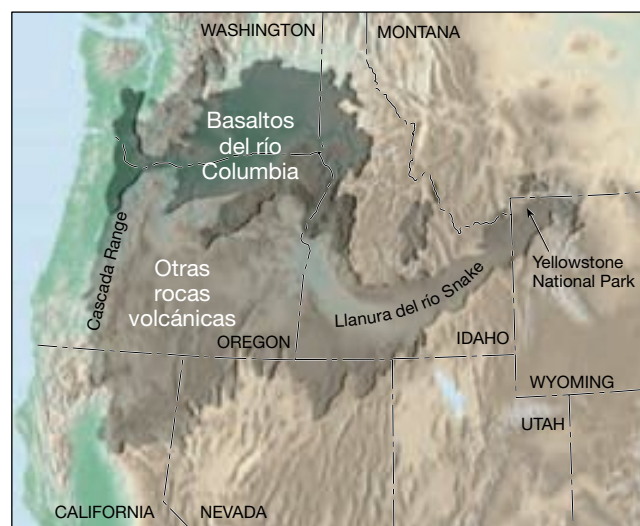
▲ Figura 5.14 Áreas volcánicas que forman la llanura de Columbia en el Pacífico noroccidental. Los basaltos del río Columbia cubren un área de casi 200.000 kilómetros cuadrados. La actividad empezó aquí hace unos 17 millones de años conforme la lava salió de grandes fisuras, acabando por producir una llanura basáltica (plateau) con un grosor medio de más de un kilómetro. (Tomado de U. S. Geological Survey.)
